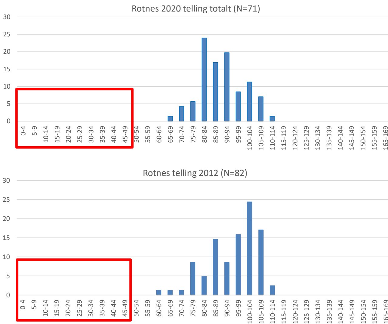
Figur 14. Lengdefordeling, vist som prosentandel av lengdeklasser i mm, av alle levende elvemuslinger i telling på stasjon Rotnes i Nitelva i 2012 (N=82) og 2020 (N=71). Rød markering viser rekruttering av muslinger.
