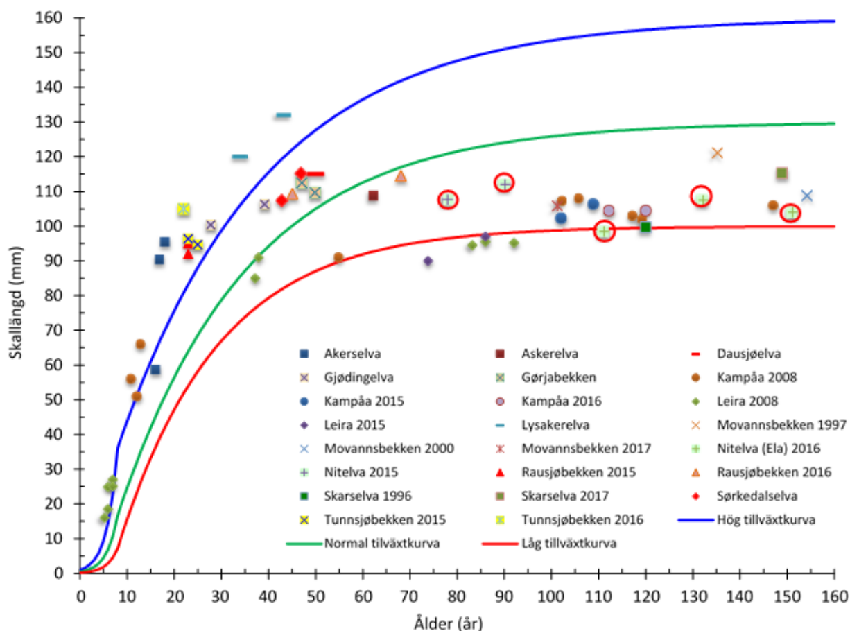
Figur 16. Figuren viser forholdet mellom alder og skallengden, og de tre normale vekstkurvene for elvemuslingen i Norden, lav vekst, normal vekst og høy vekst (Meret og Sandaas u/arb.). Nitelva er markert med røde sirkler på kurven for lav vekst. Juvenile muslinger fra Nitelva har i dag høy vekst, men den avtar med alderen.
