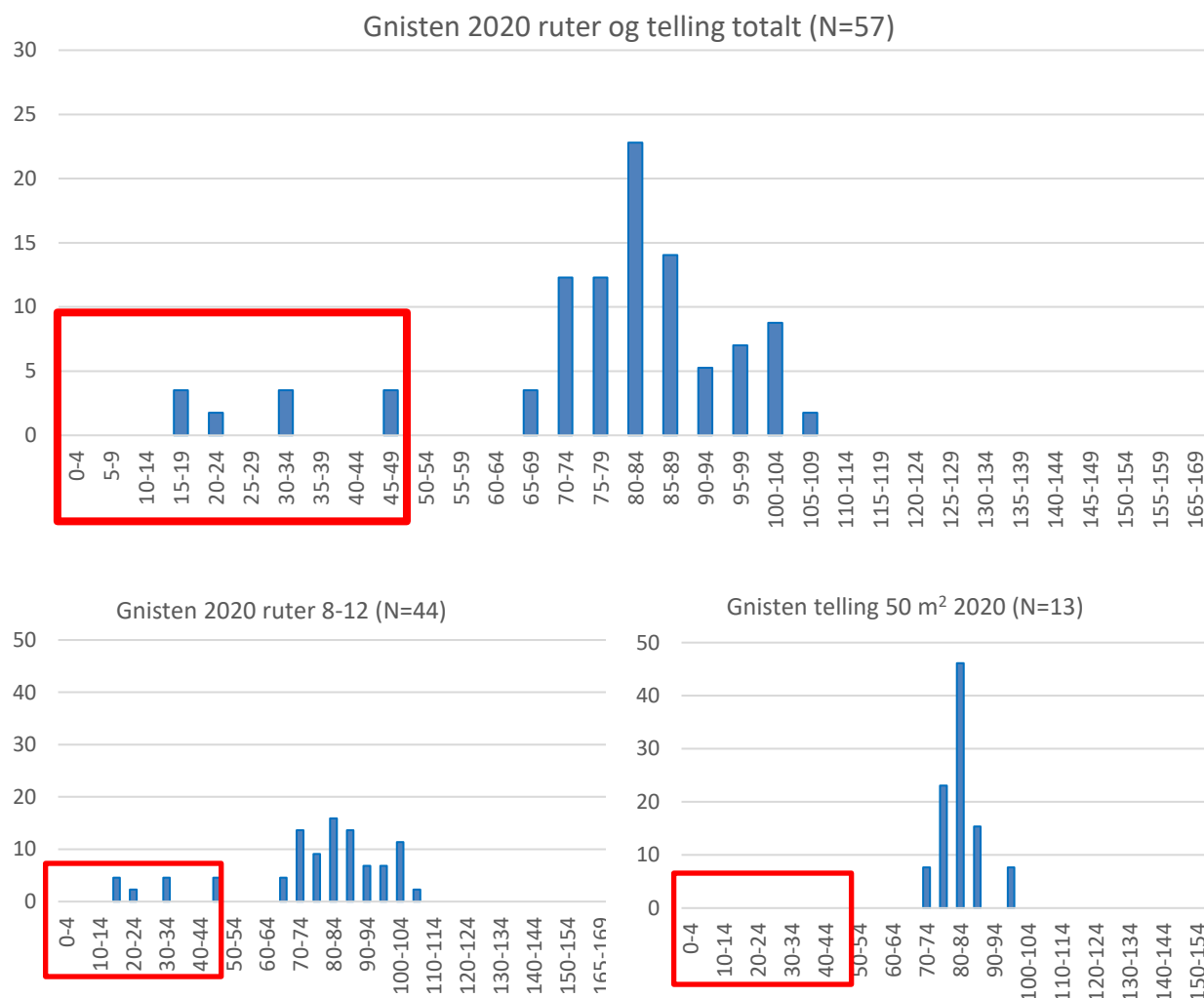
Figur 11. Lengdefordeling, vist som prosentandel av lengdeklasser i mm, av alle levende elvemuslinger, samt for graveruter og telling, på stasjon Gnisten i Nitelva i 2020. Rød markering viser rekruttering av muslinger.
